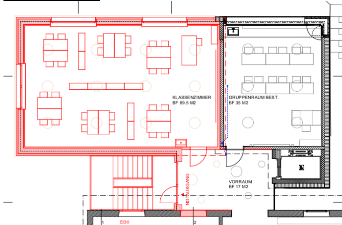
Grundriss 1.OG:
