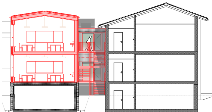
Schnitt:
