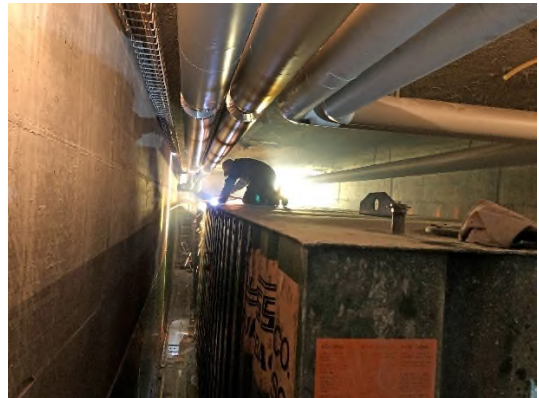
Impressionen vor und nach der Demontage der Tanks
